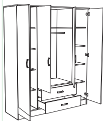
Ormar Iva 4K2F Wardrobe "Iva 4K2F" 163,5 x 53 x 200 cm
