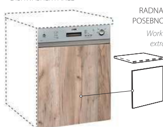
IN MASKA 60 x 60 60 x 60 x 1,8 cm ID KMAS 6060**
