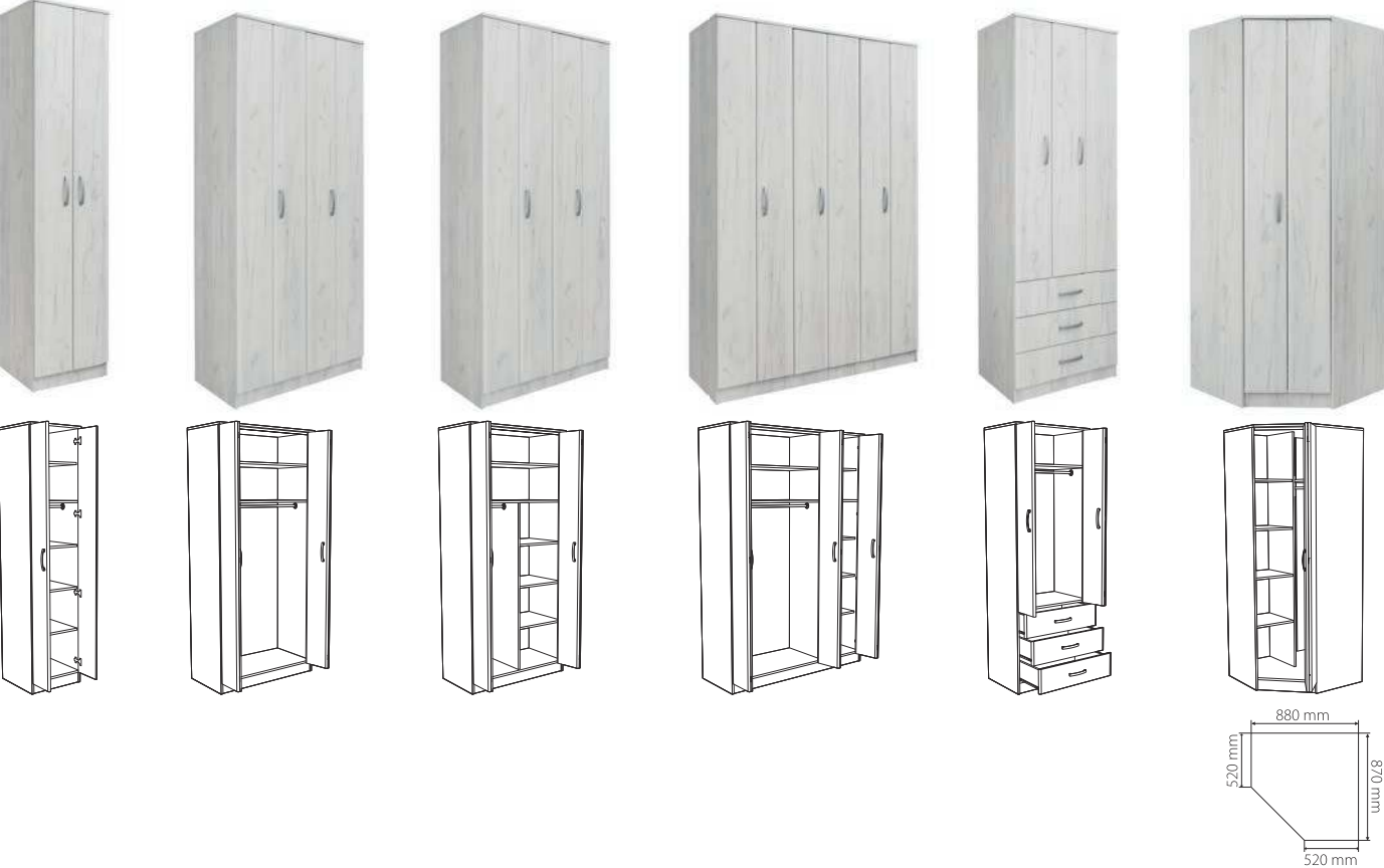
F1 • 50 x 52 x 222 cm ID 3040** F2 • 100 x 52 x 222 cm ID 3041** F2 POL • 100 x 52 x 222 cm ID 3042** F3 • 150 x 52 x 222 cm ID 3043** F75 • 75 x 52 x 222 cm ID 3045** FU • 88/52 x 87/52 x 222 cm ID 3046**
