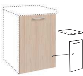
IN MDF MASKA 45 x 72 45 x 72 x 1,8 cm ID KMAS 4572**
