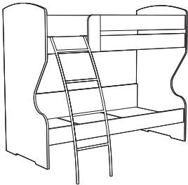
Krevet na sprat/Bunk bed 205 x 96,4 x 173,5 cm ID J492309
